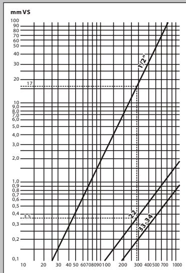
Wykres strat ciśnienia
